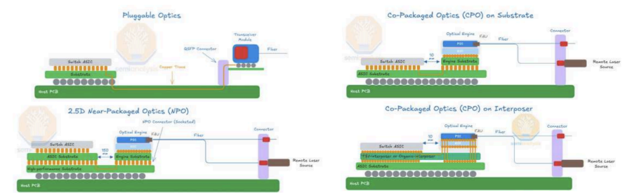
图：可插拔光模块、NPO、CPO示意图
